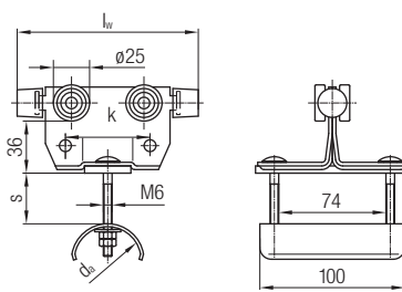
Kabelový vozík
