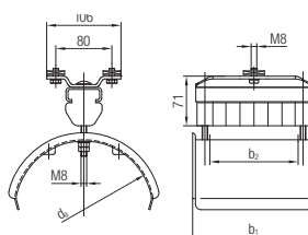
Koncová svorka
