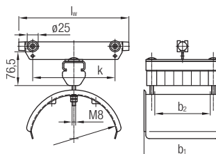
Kabelový vozík
