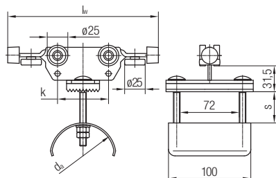
Kabelový vozík
