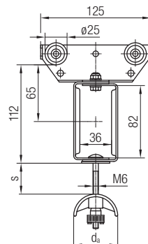
Unášecí vozík
