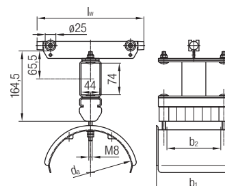
Unášecí vozík
