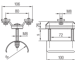
Koncová svorka
